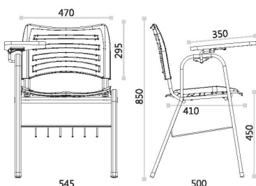
FIT UNIVERSITÁRIA PRANCHETA ESCAMOTEÁVEL *LADO DIREITO / LADO ESQUERDO
