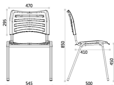
FIT 4 PÉS EMPILHÁVEL
