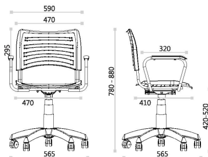
FIT GIRATÓRIA COM BRAÇO
