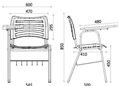
FIT UNIVERSITÁRIA PRANCHETA FIXA *LADO DIREITO / LADO ESQUERDO
