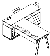
MESA GERENTE C/ ARMARIO CREDENZA LD
